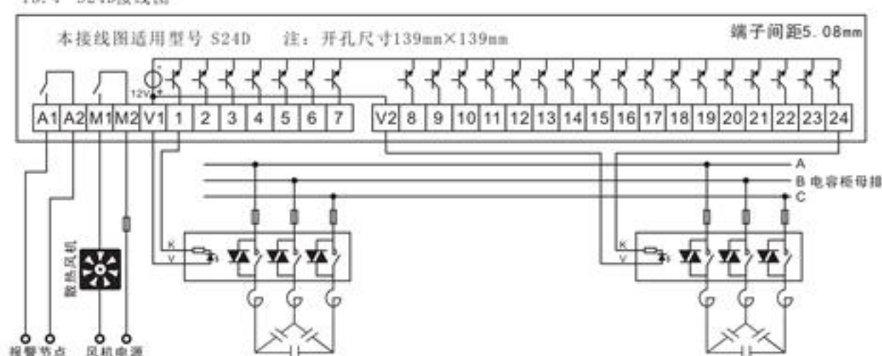
13.4 S24D接线图
