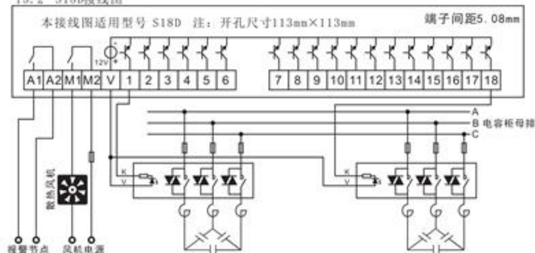
13.2 S18D接线图
