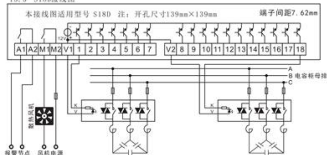
13.3 S18D接线图
